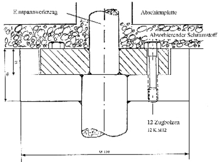
Abbildung 10.1 Schematische Darstellung des Zwischenstücks
