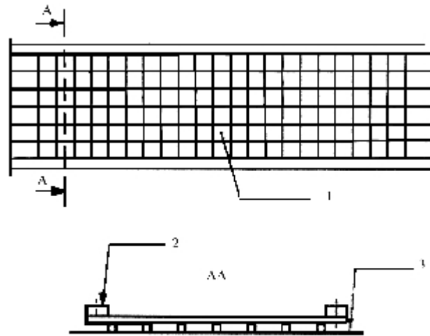
Abbildung 39.2 Ausführungsdetail und Montage der Laufbahn
