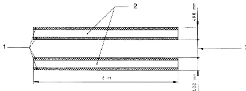
Abbildung 39.1 Schema der Prüfstrecke
