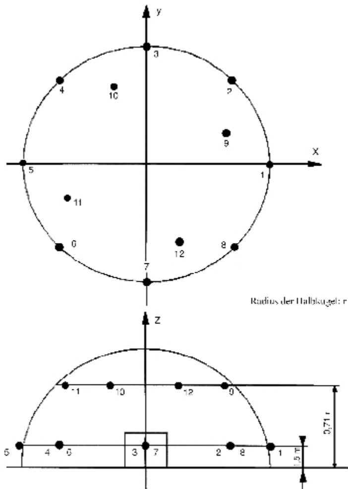
Abbildung Zusätzliche Anordnung von Mikrofonen auf der halbkugelförmigen Messfläche (12 Mikrofonpositionen)
